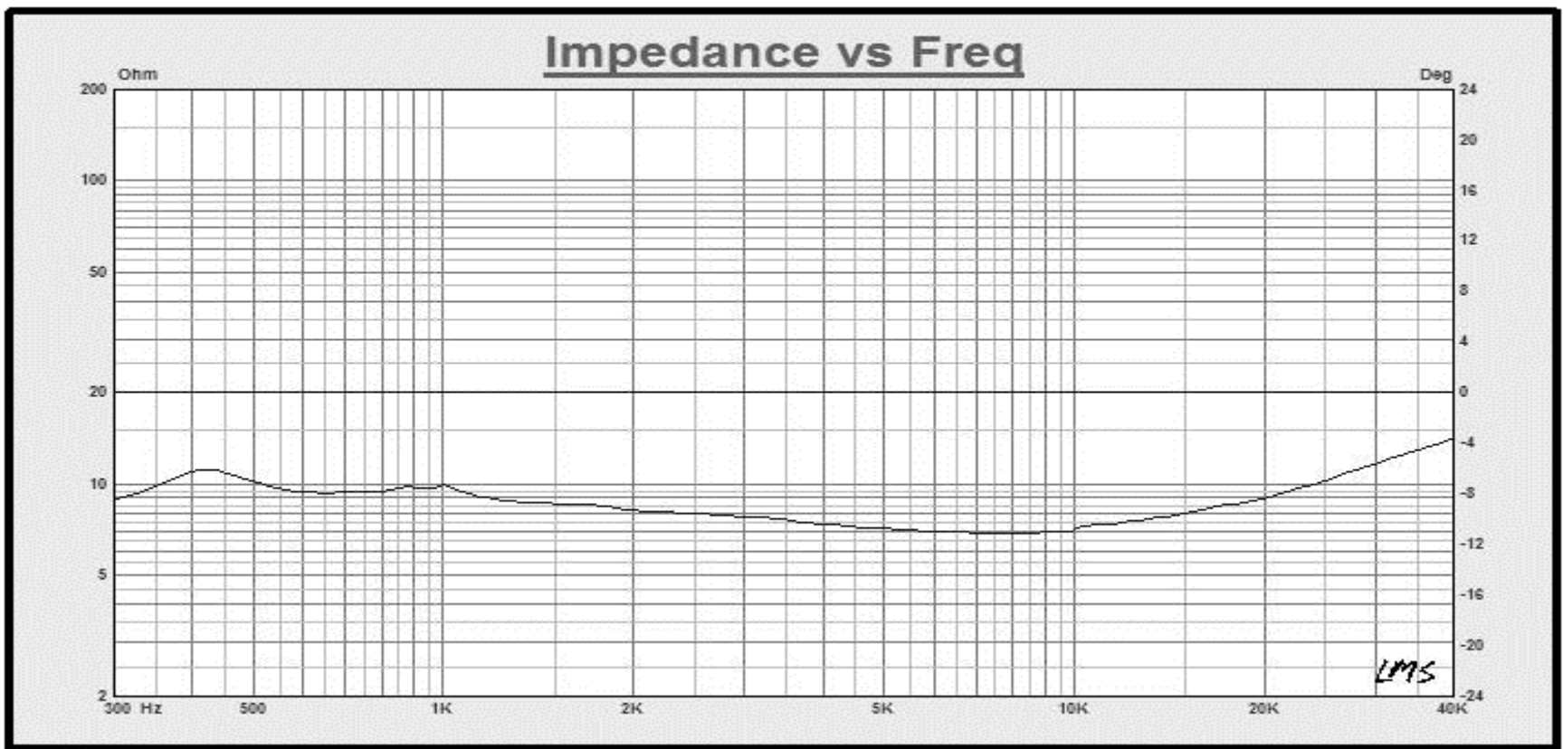
图 2 CQ76-2H LMS 阻抗曲线图
