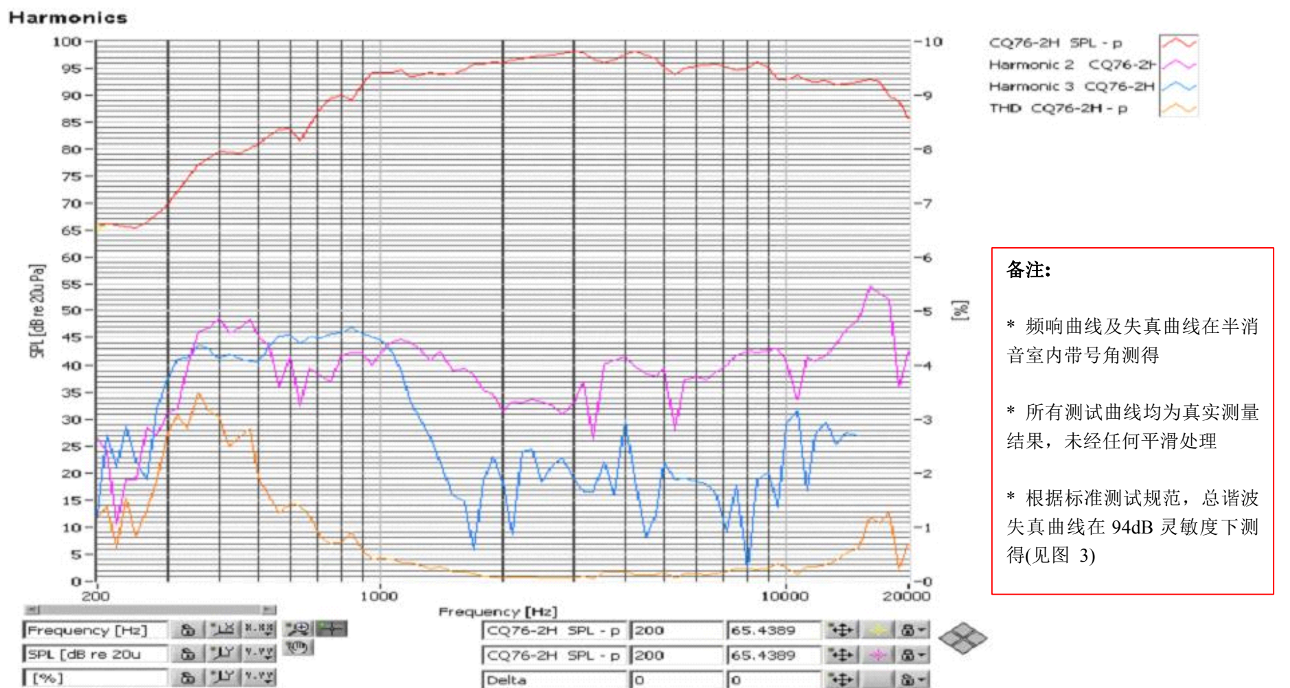
图 3 CQ76-2H Soundcheck 总谐波失真及 2 次、3 次谐波失真曲线图
