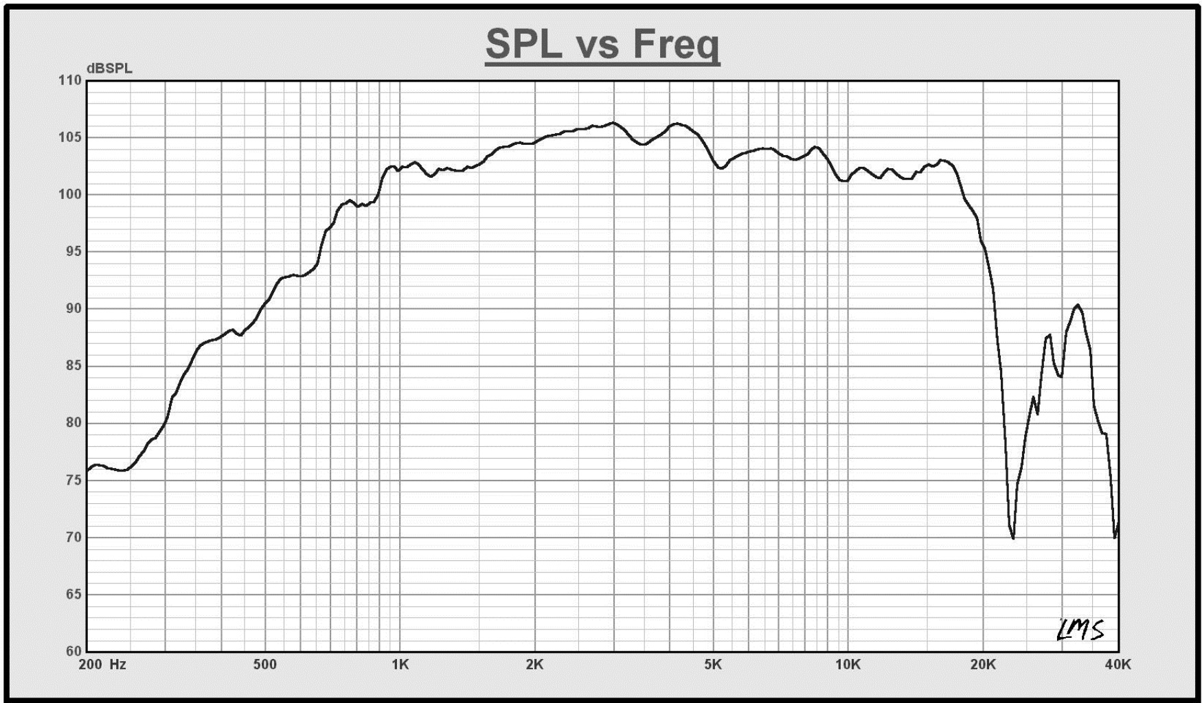
图 1 CQ76-2H LMS 频响曲线图
