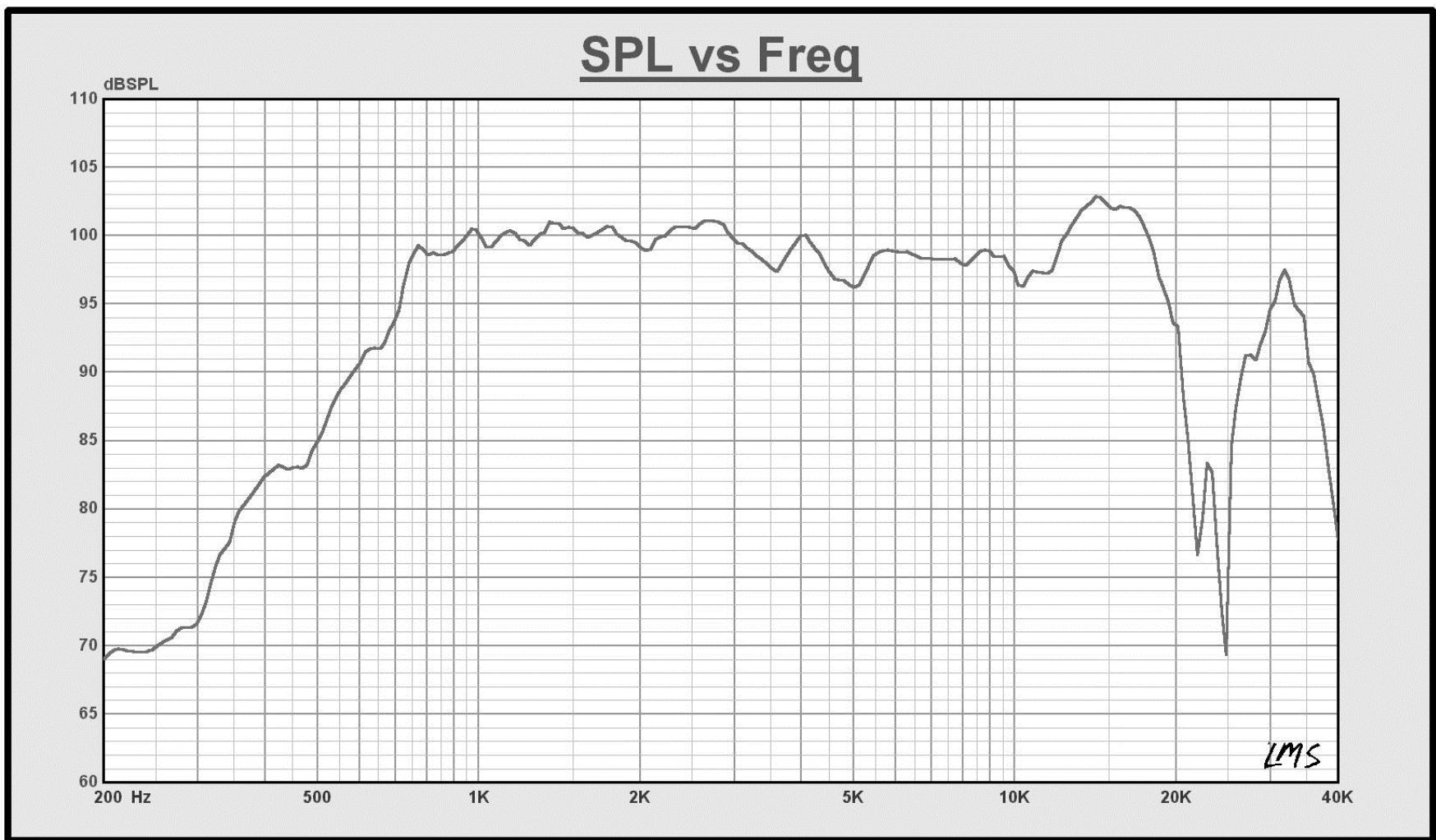
图 1 CQ76-H LMS 频响曲线图
