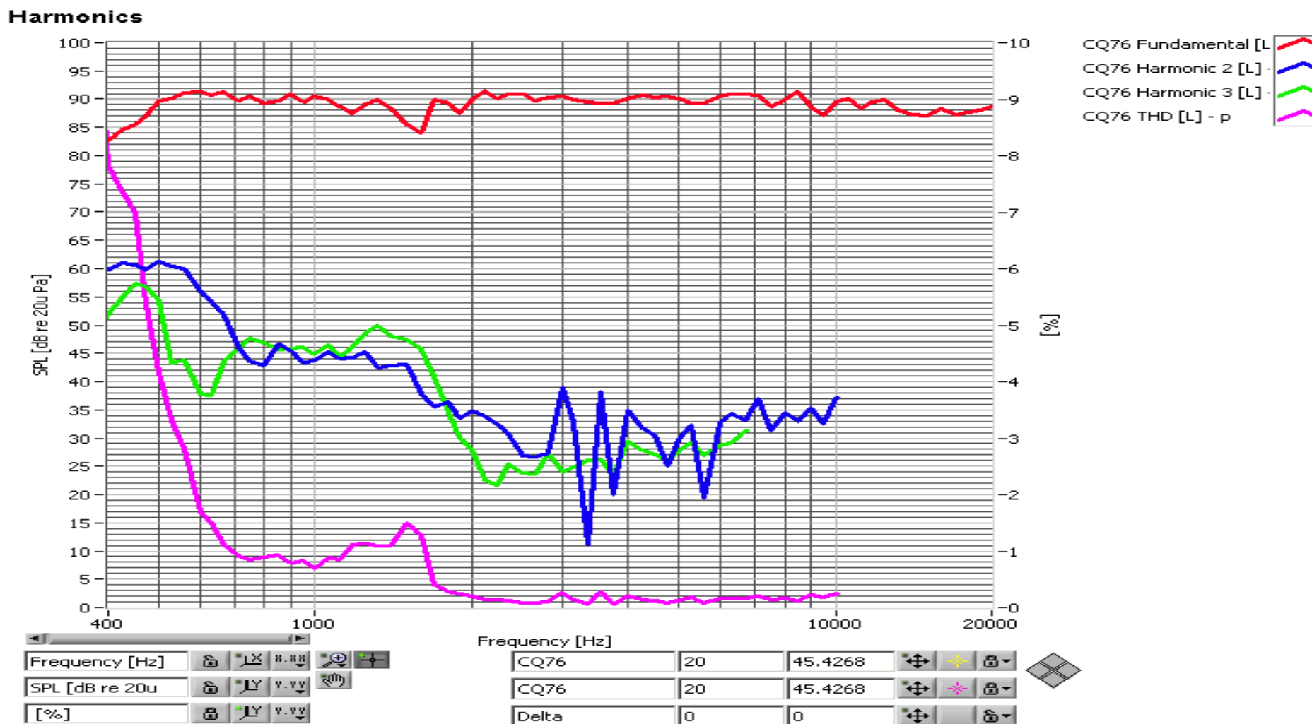
图2 CQ76 SoundCheck 频响曲线
