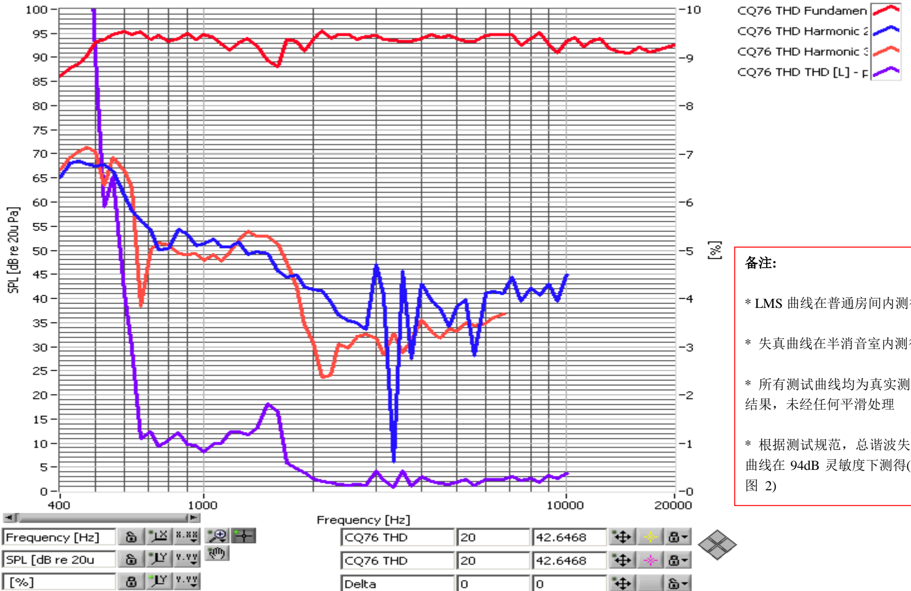
图 3 CQ76 Soundcheck 总谐波失真及 2 次、3 次谐波失真曲线图
