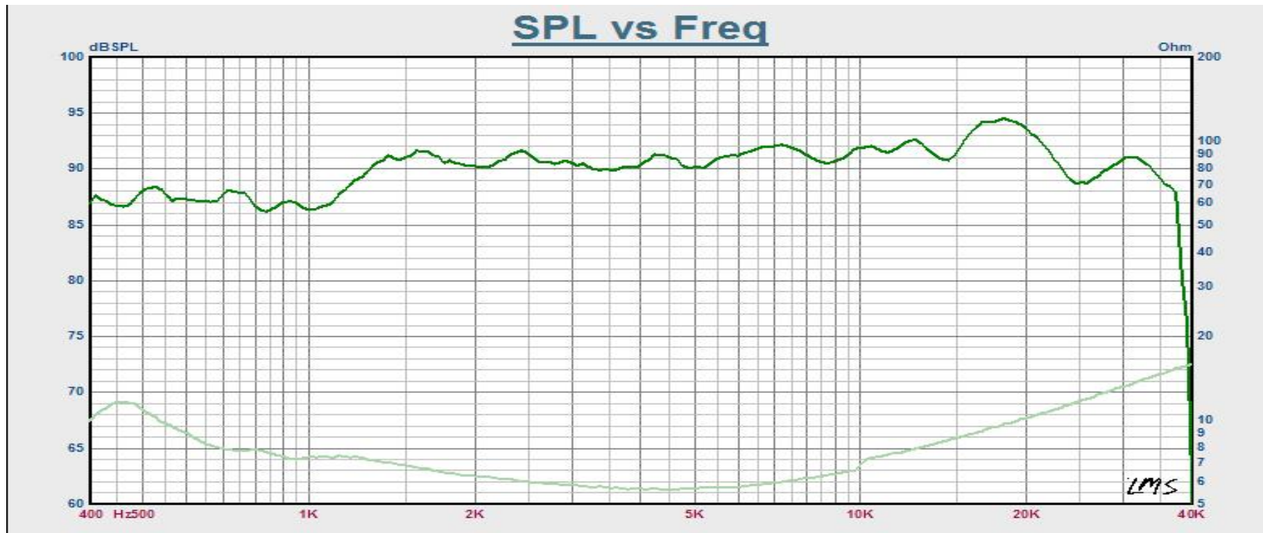
图1 CQ76 LMS 频响及阻抗曲线
