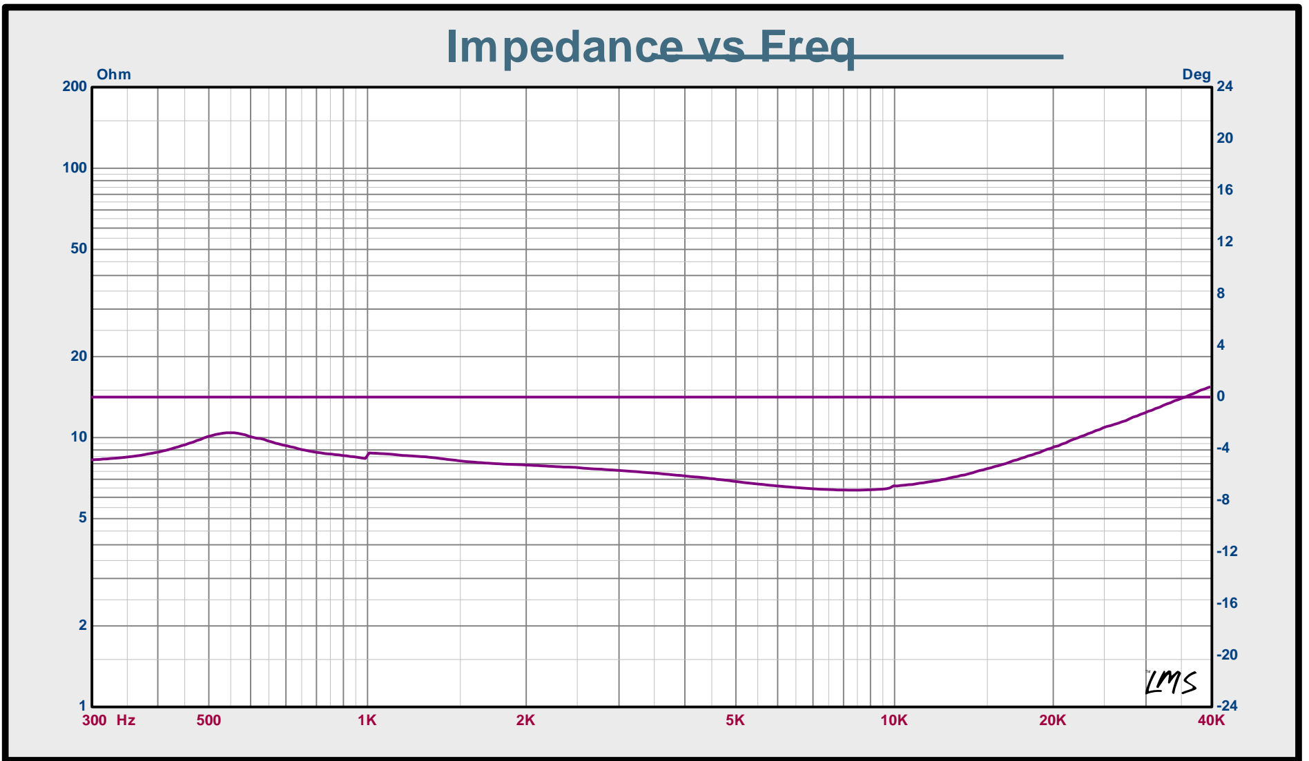
图 1. 阻抗曲线
