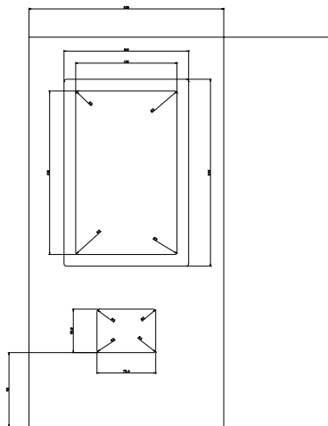
3. 音箱后视图 Box Back View
